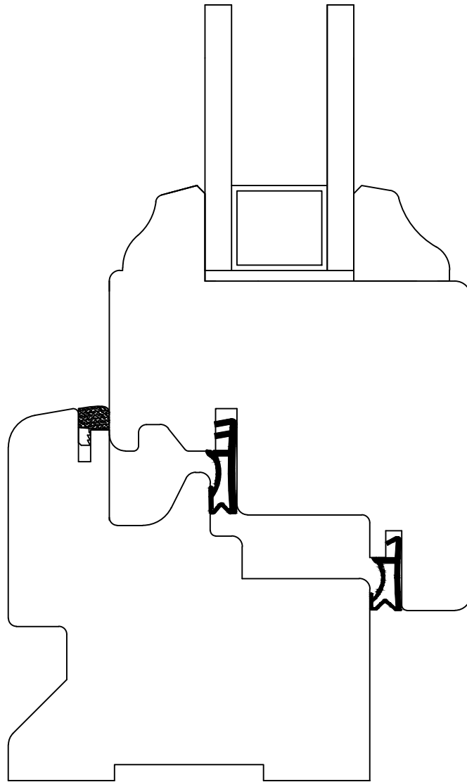
Legno 68 mm basic - profilo centro storico -
