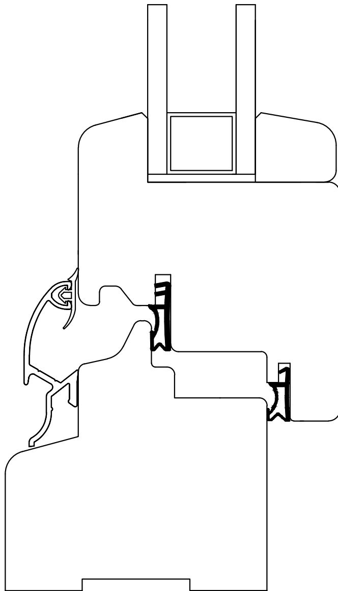
Legno 68 mm basic - profilo standard -
